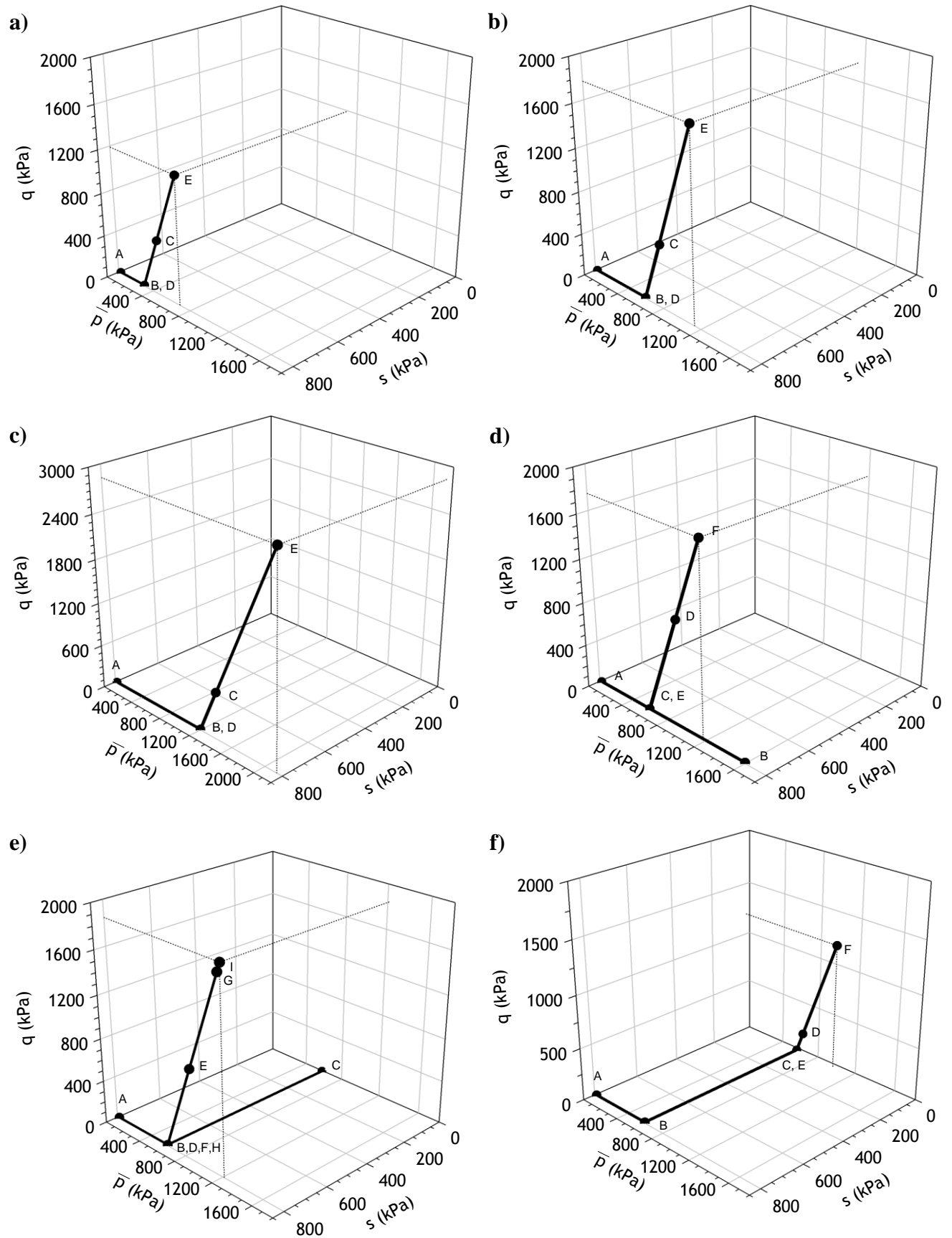
Fig. 3. Stress paths for suction-controlled triaxial tests: (a) IS-OC-03; (b) IS-NC-06; (c) IS-NC-12; (d) IS-OC-06; (e) IWS-OC-01; (f) IWS-NC-02.
